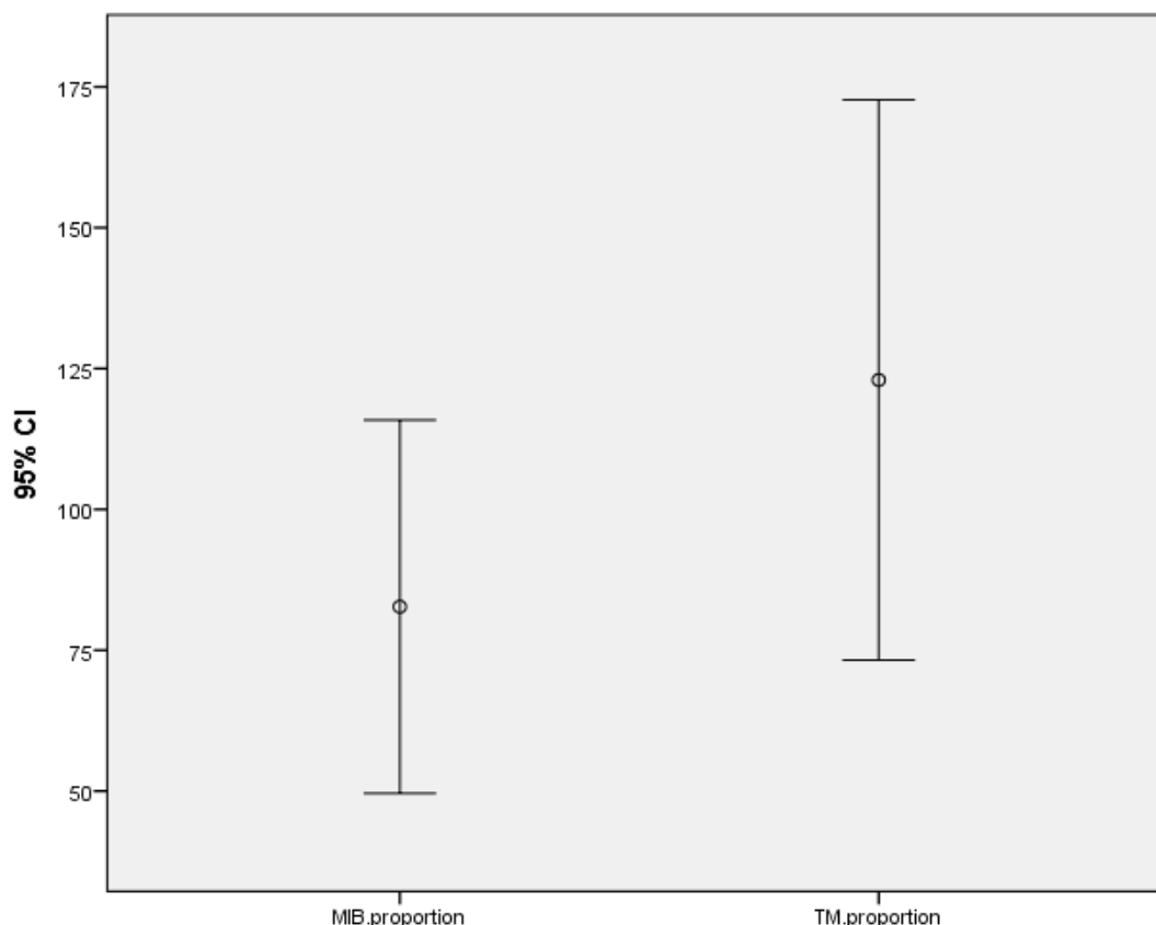
نمودار شماره ۲: مقایسه ی بازه ی تغییرات تناسب نیرو به محیط در روکش های 3M و MIB
